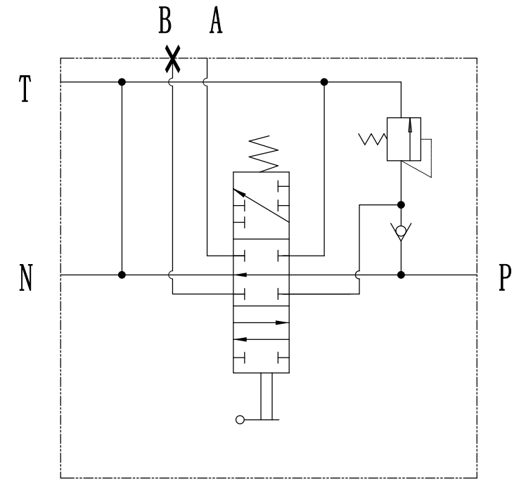
液压原理图
