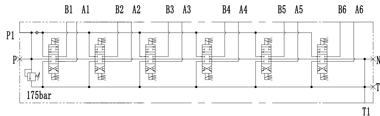
原理图
