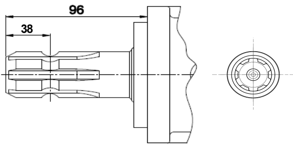
1"-3/8 DIN 9611 -Z6
