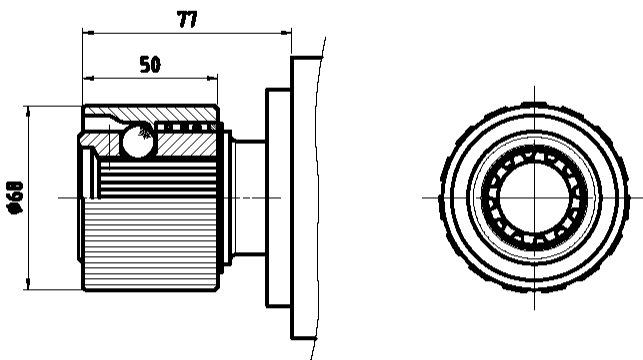
1"-3/8 DIN 9611 -Z21
