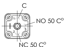
Схема включения
