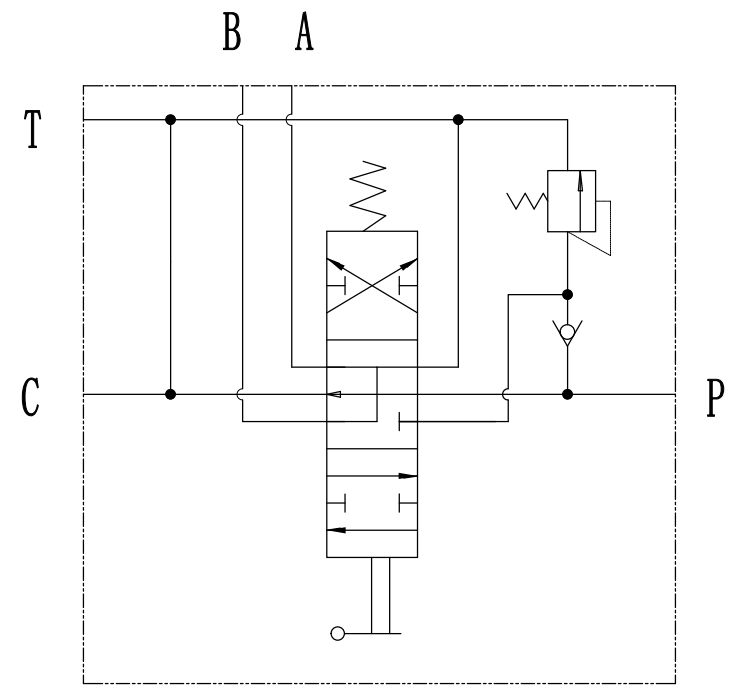
液压原理图
