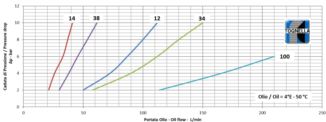
FT 270/5 PORTATA FLUSSO LIBERO / FREE FLOW
