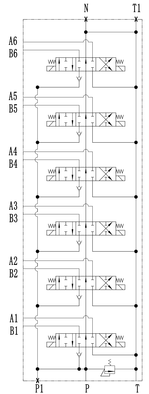
液压原理图
